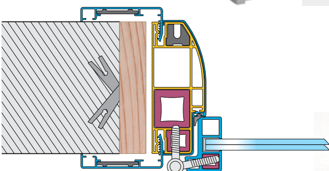
PARTICOLARE SEZIONE TELAIO
