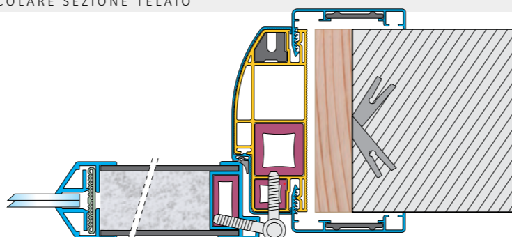
PARTICOLARE SEZIONE TELAI
