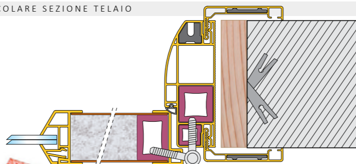
PARTICOLARE SEZIONE TELAIO
