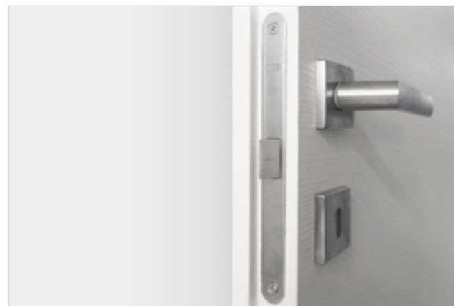
Serratura con scrocco e mandata
